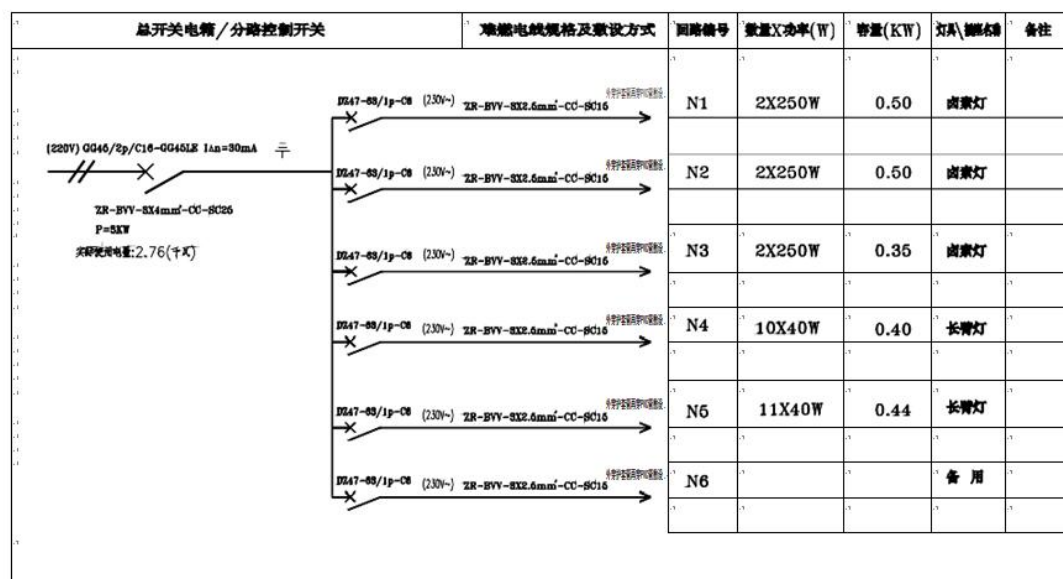
配电系统图
