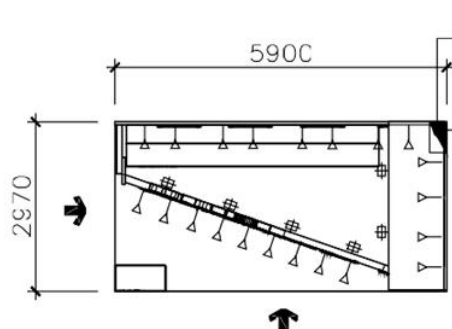
电气平面图
